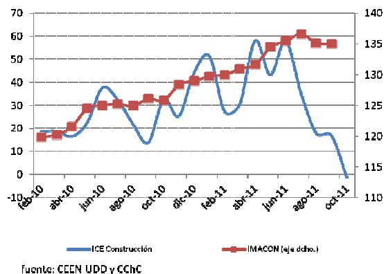
Gráfico 2 ICE Construcción e Imacon (Índice centrado en cero e Índice)
